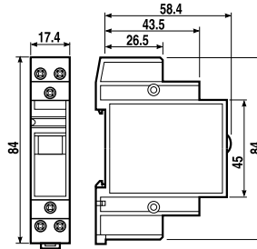
Тип 22.24 Винтовой клеммы
