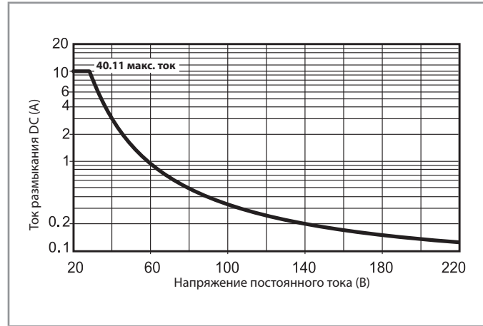
Н 40.2 - Макс. отключающая способность DC1 Тип 40.11
