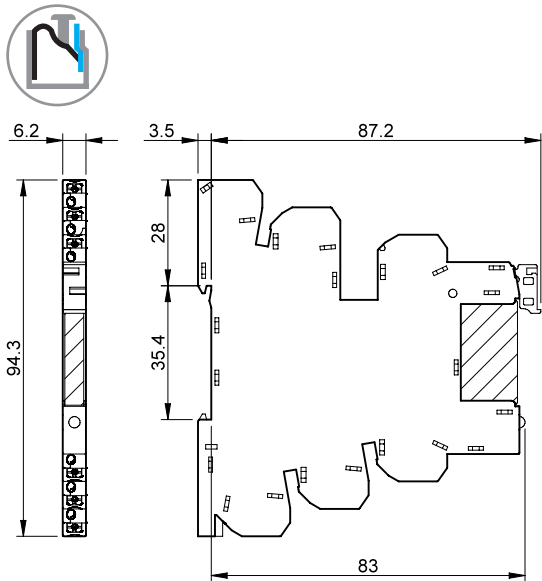
Тип 39.70 39.71 Клеммы Push-in
