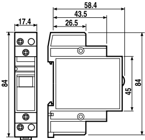
Тип 22.23 Винтовой клеммы
