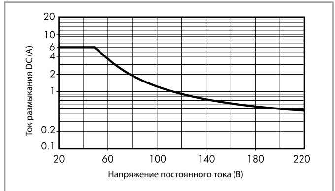
H 7S14* - Макс. отключающая способность DC - 7S.14/34
