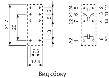
Вид сбоку
