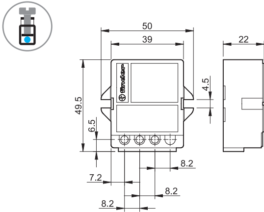
Тип 15.51 Винтовой клеммы
