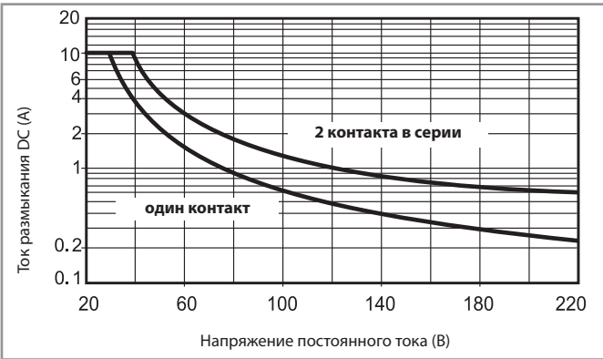
Н 40.6 - Макс. отключающая способность DC1 Тип 40.62
