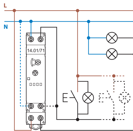
4-проводное соединение
