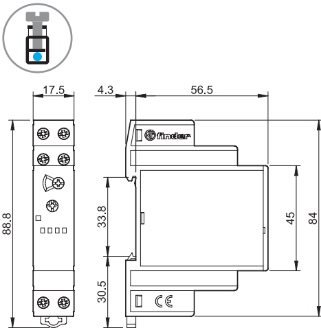
Тип 13.61 Винтовые клеммы
