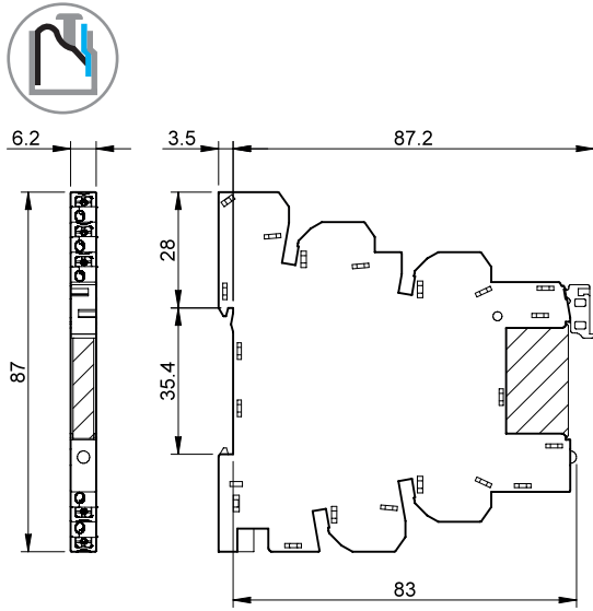
Тип 39.00/39.01 39.50/39.51 Клеммы Push-in
