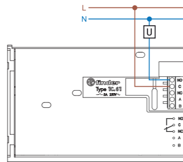
Схема подключения
