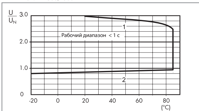
R 67-3 - Отношение рабочего диапазона к температуре окр. среды, 67.xx-x300/x500
